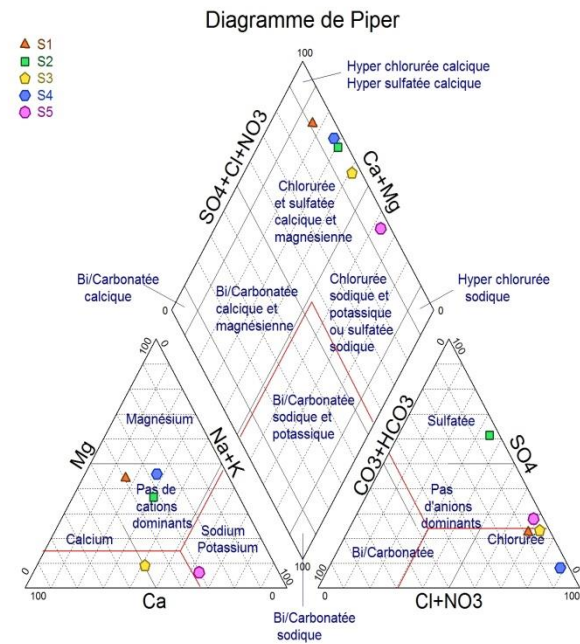
Figure 1 : Diagramme de Piper
