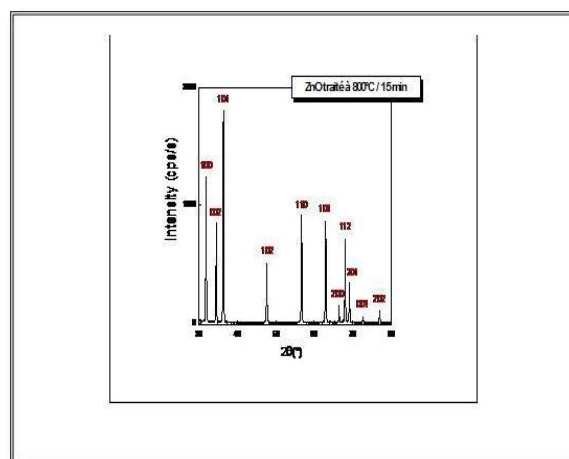
Figure 1. Diagramme de diffraction des rayons X de la poudre ZnO, CoK \alpha 1 ( \lambda=1.789 \text{ \AA} ) (Bouloudenine, 2006)
